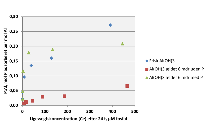
Figur 2. Binding af P til frisk og 6 mdr. gammel Al(OH) 3 ved udrystning i forskellige fosfatopløsninger i 24 timer. X-aksen viser ligevægtskoncentrationen (C e ) efter udrystning og Y-aksen viser adsorptionen af fosfat-P til Al(OH) 3 .
